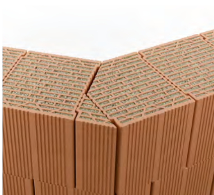
2. Mauerwerksschicht 30 cm
