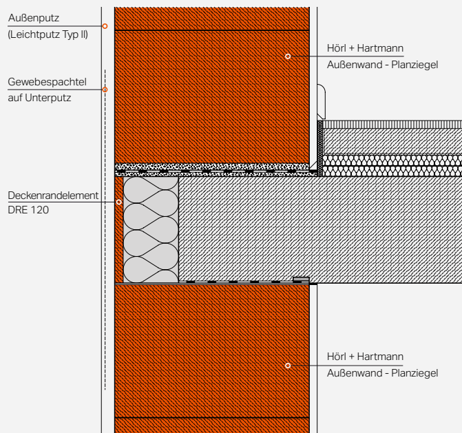
Einbau als Deckenrandelement
