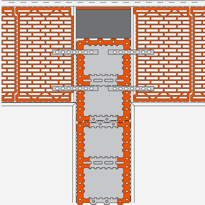
Außenwand mit 42,5er UNIPOR CCORISO oder SILVACOR Ziegel
