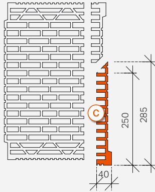
3. Scheibe absägen
