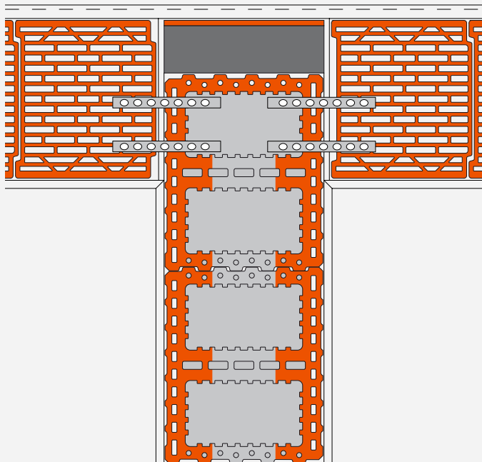
Außenwand mit 30er UNIPOR CORISO oder SILVACOR Ziegel
