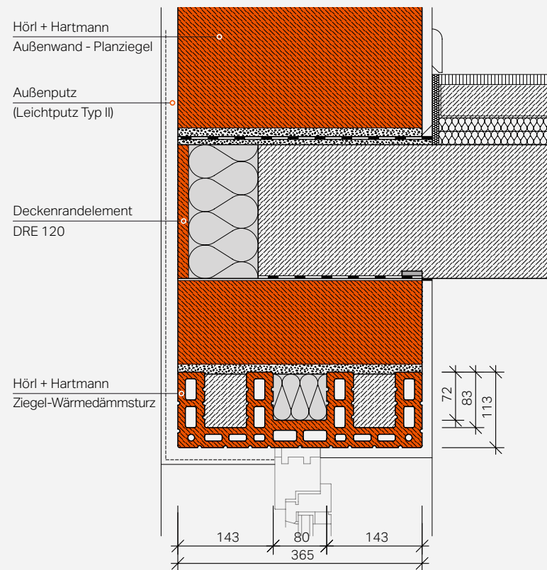
Einbindung eines Ziegel-Wärmedämmsturzes mit Höhen- ausgleichsziegel (HAZ) und Ziegel-Wärmedämmsturz
