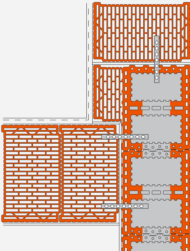
Abknickende Außenwand mit gefülltem 42,5er UNIPOR Ziegel
