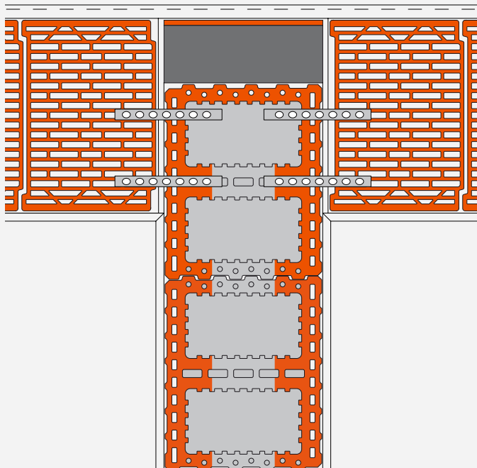
Außenwand mit 36,5er UNIPOR CORISO oder SILVACOR Ziegel
