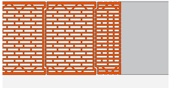
HALBER VERSTÄRKTER LAIBUNGSZIEGEL
