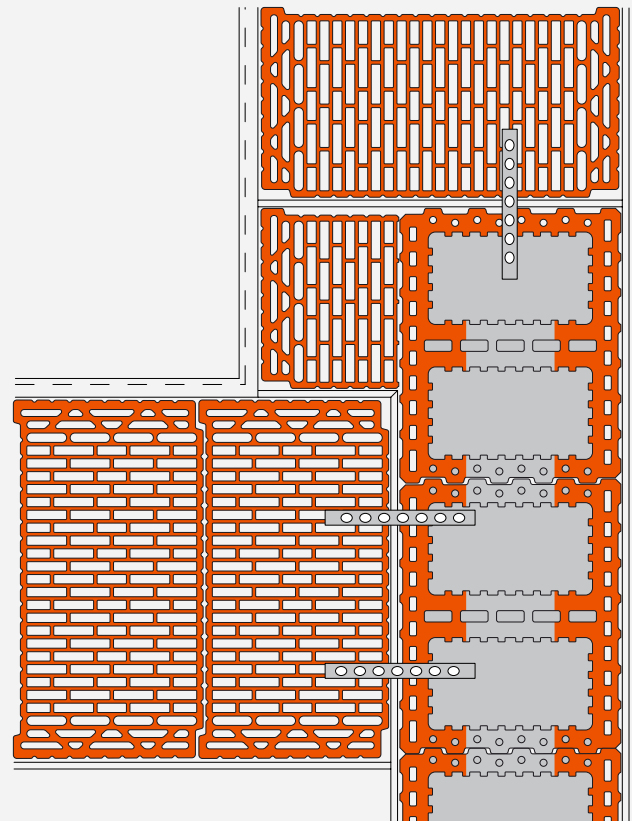
Abknickende Außenwand mit gefülltem 49er UNIPOR Ziegel
