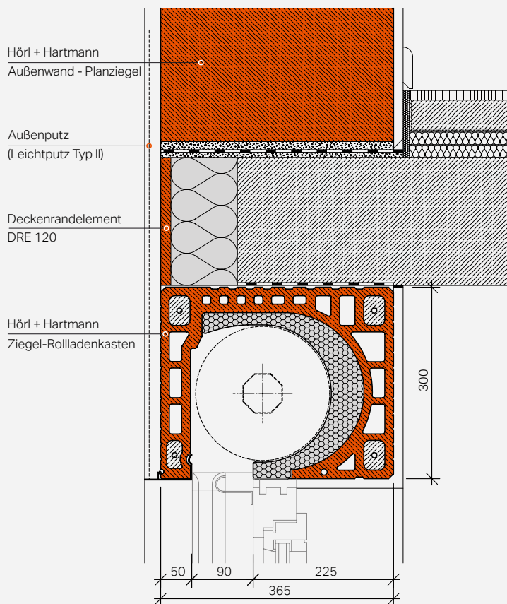
Einbindung eines Ziegel-Rolladenkastens anstelle eines Fenstersturzes
