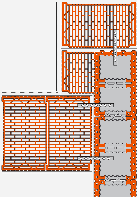
Abknickende Außenwand mit gefülltem 42,5er UNIPOR Ziegel
