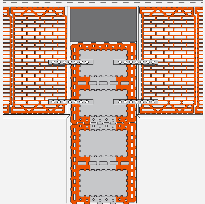
Außenwand mit 49er UNIPOR CORISO oder SILVACOR Ziegel
