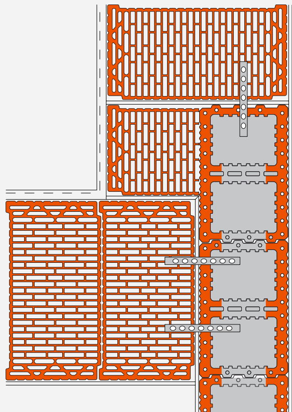
Abknickende Außenwand mit gefülltem 49er UNIPOR Ziegel
