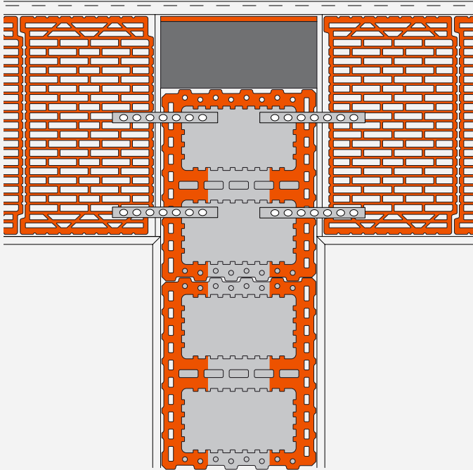
Außenwand mit 42,5er UNIPORCORISO oder SILVACOR Ziegel
