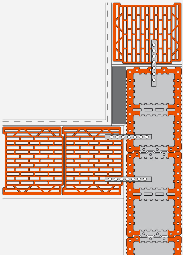
Abknickende Außenwand mit gefülltem 30er UNIPOR Ziegel
