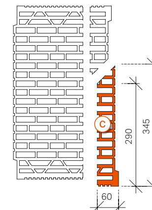
3. Scheibe absägen
