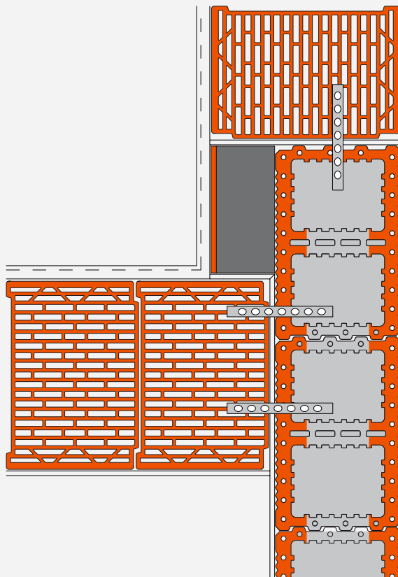
Abknickende Außenwand mit gefülltem 36,5er UNIPOR Ziegel
