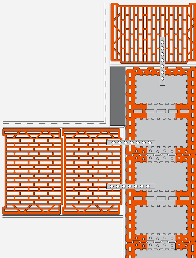
Abknickende Außenwand mit gefülltem 36,5er UNIPOR Ziegel
