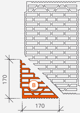
2. Ecke absägen
