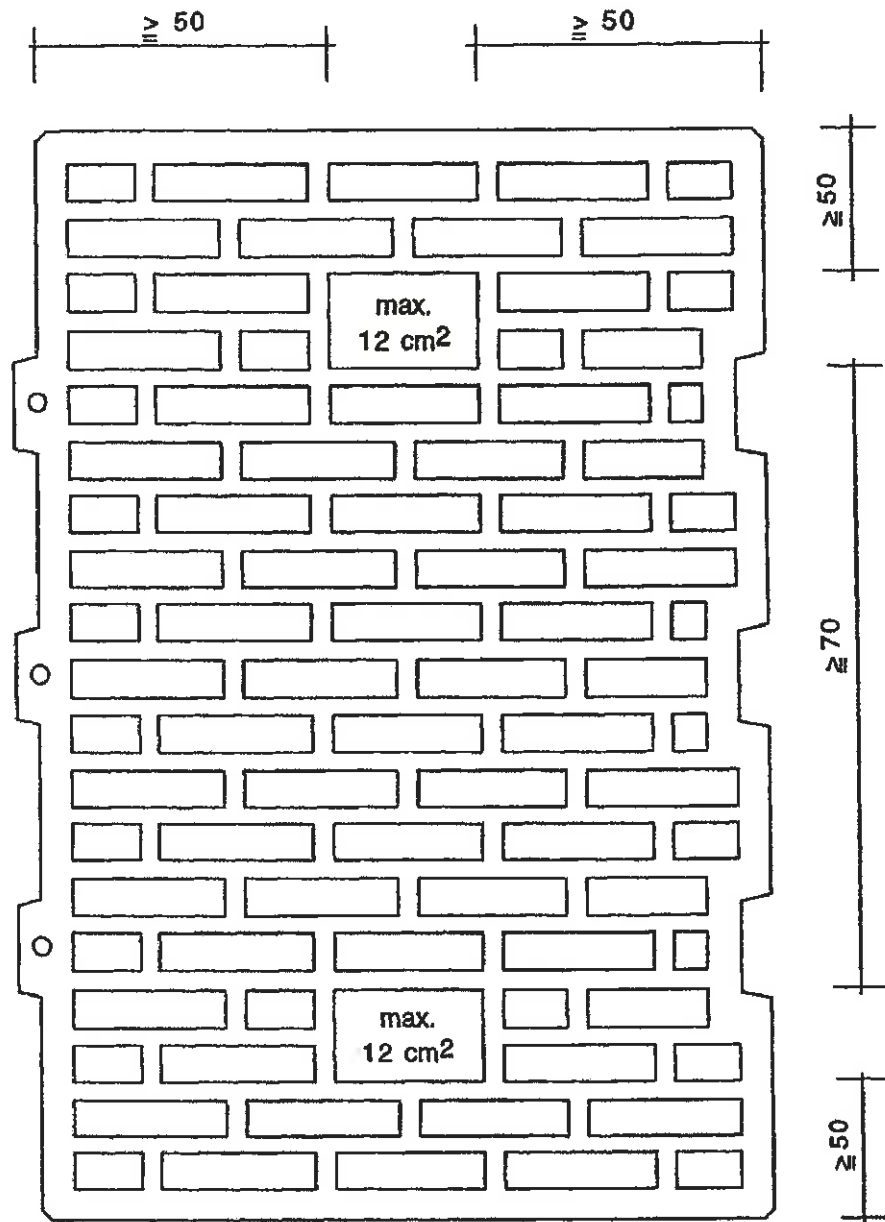
Prinzipdarstellung Griffhilfe
