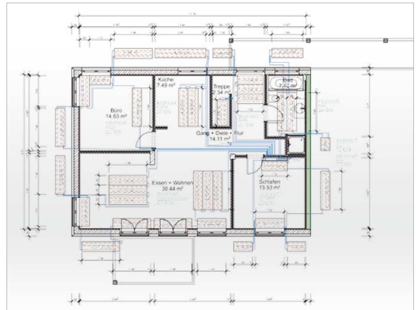
Positions- und Verlegeplan
